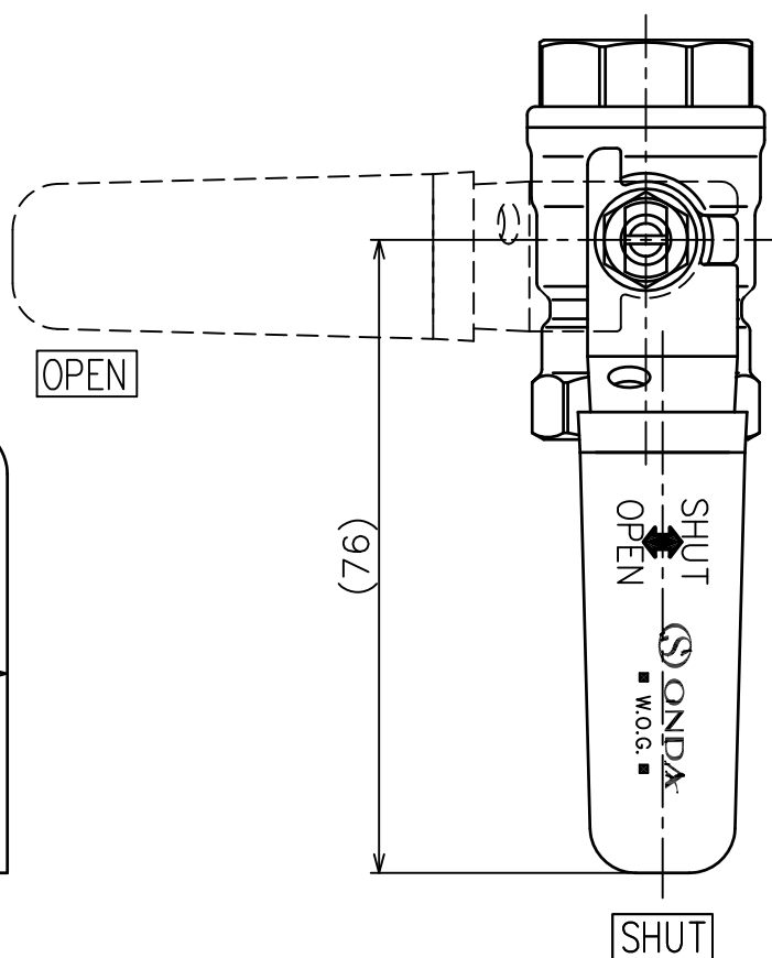
手動起動装置用ボールバルブ
